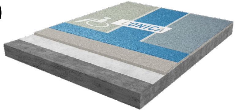
1 Primer / blocking primer optional 2 Scratch primer with QS 3 Top coat pigmented
